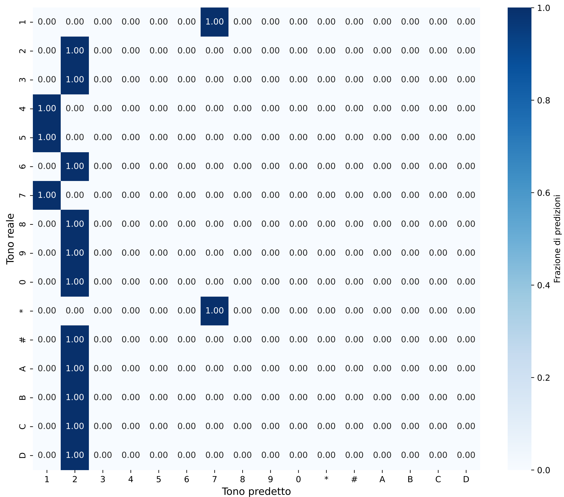
Matrice di Confusione - Singoli Toni Durata: 0.002457250711986956s
