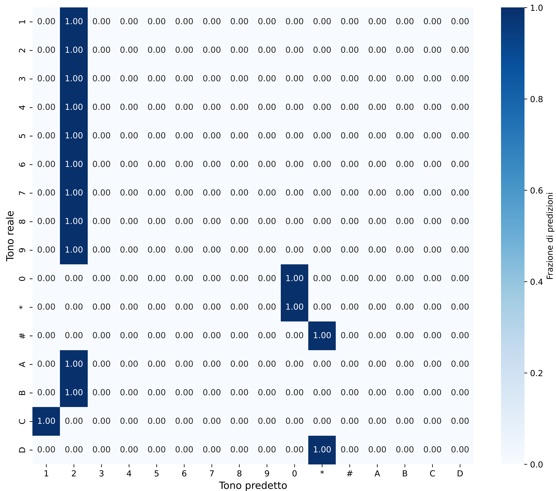
Matrice di Confusione - Singoli Toni Durata: 0.0027524625874895004s
