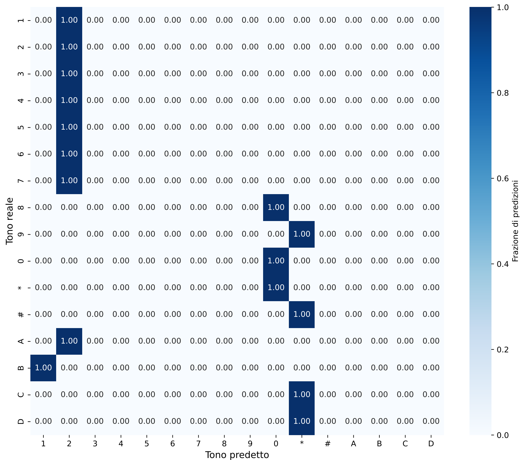
Matrice di Confusione - Singoli Toni Durata: 0.002859938296617457s
