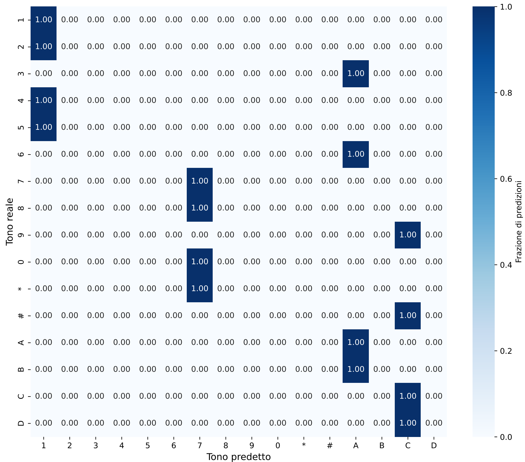
Matrice di Confusione - Singoli Toni Durata: 0.003019040530780201s
