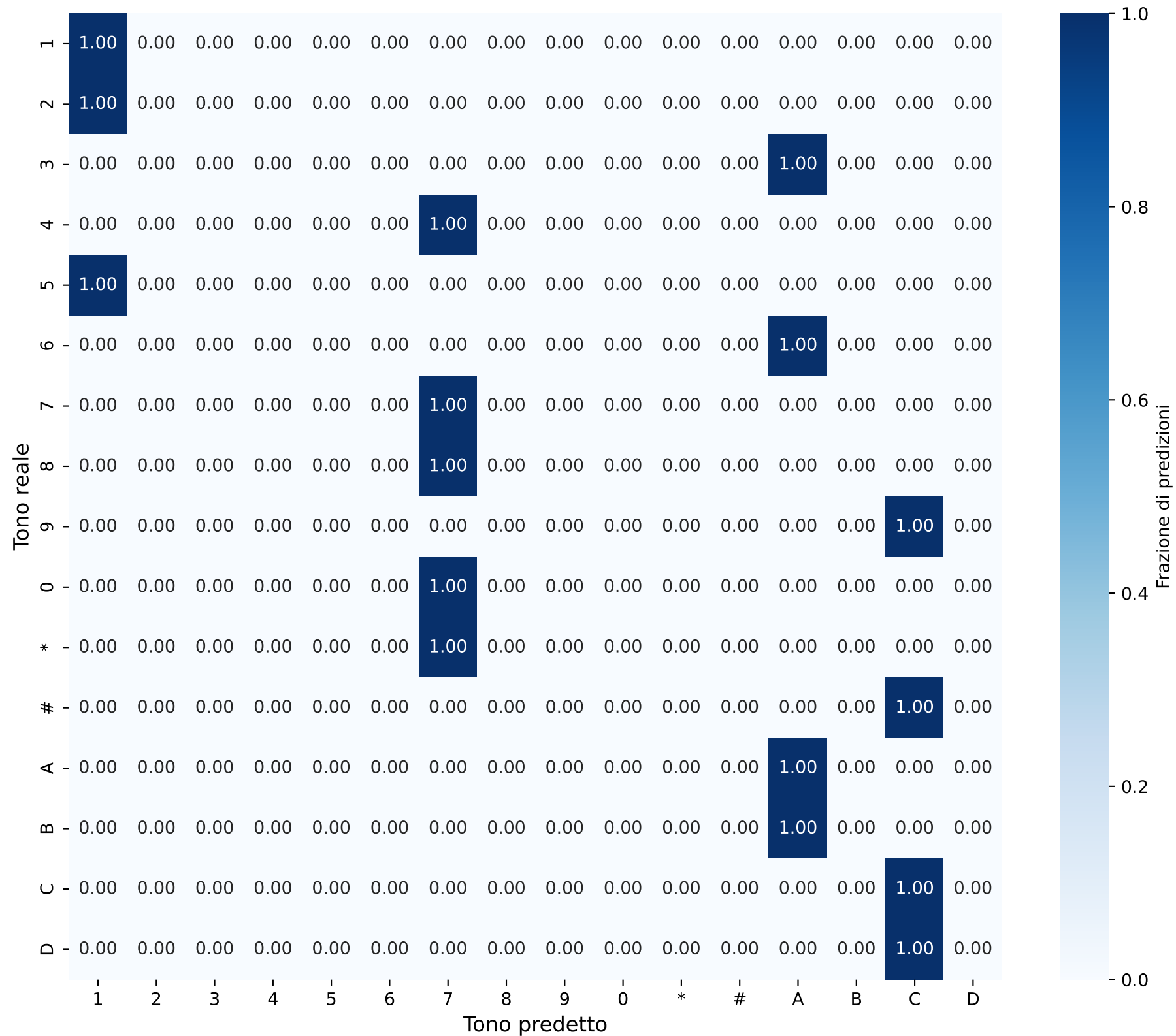
Matrice di Confusione - Singoli Toni Durata: 0.0030889042098927585s
