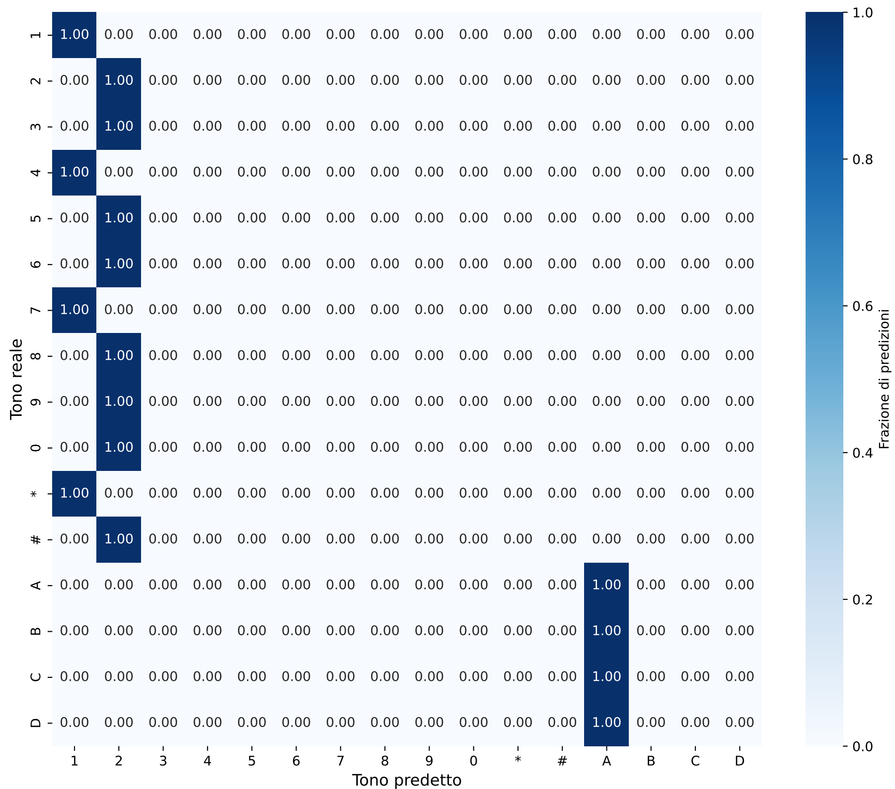
Matrice di Confusione - Singoli Toni Durata: 0.0032289932641137143s
