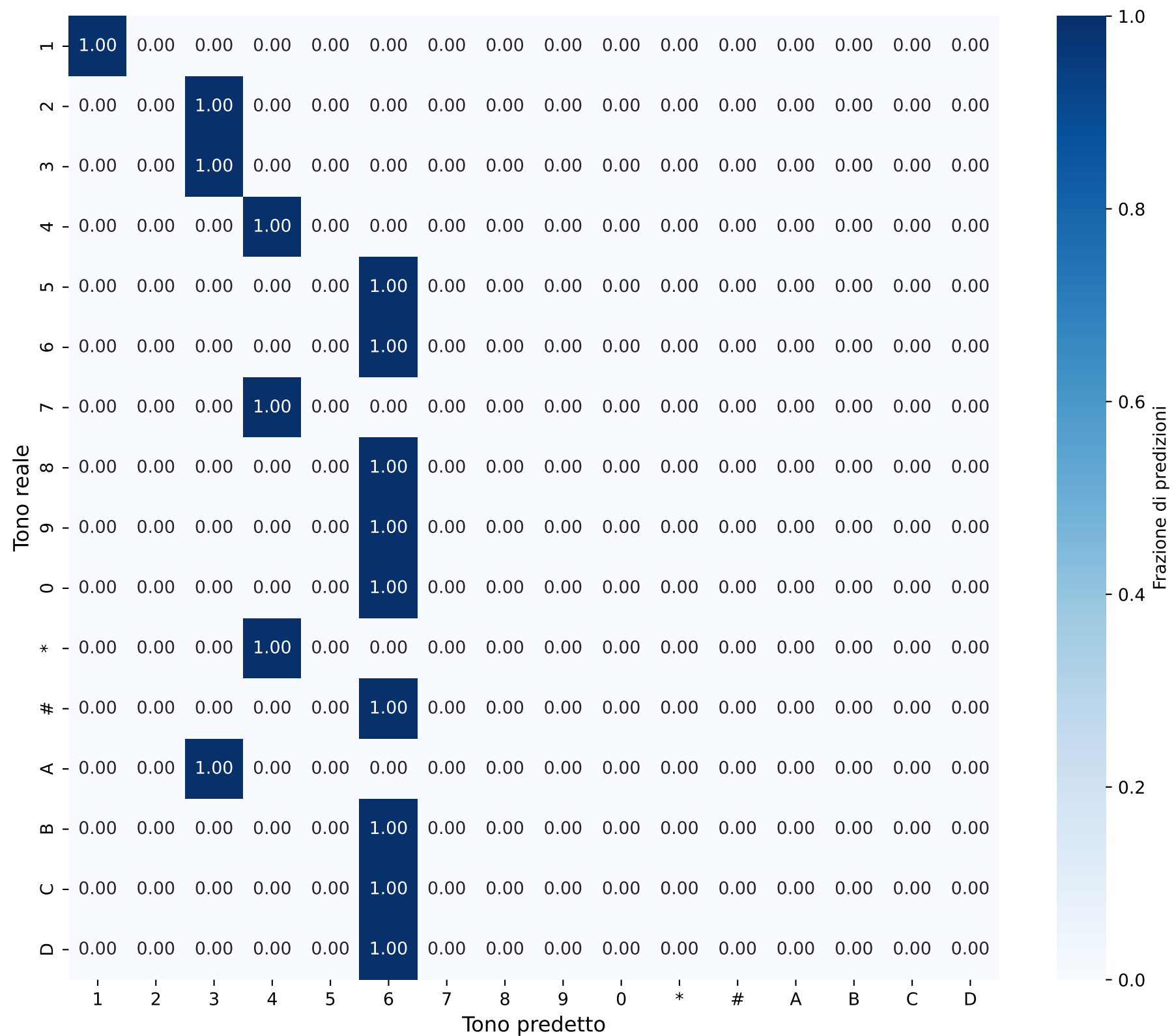
Matrice di Confusione - Singoli Toni Durata: 0.0032851692882647906s
