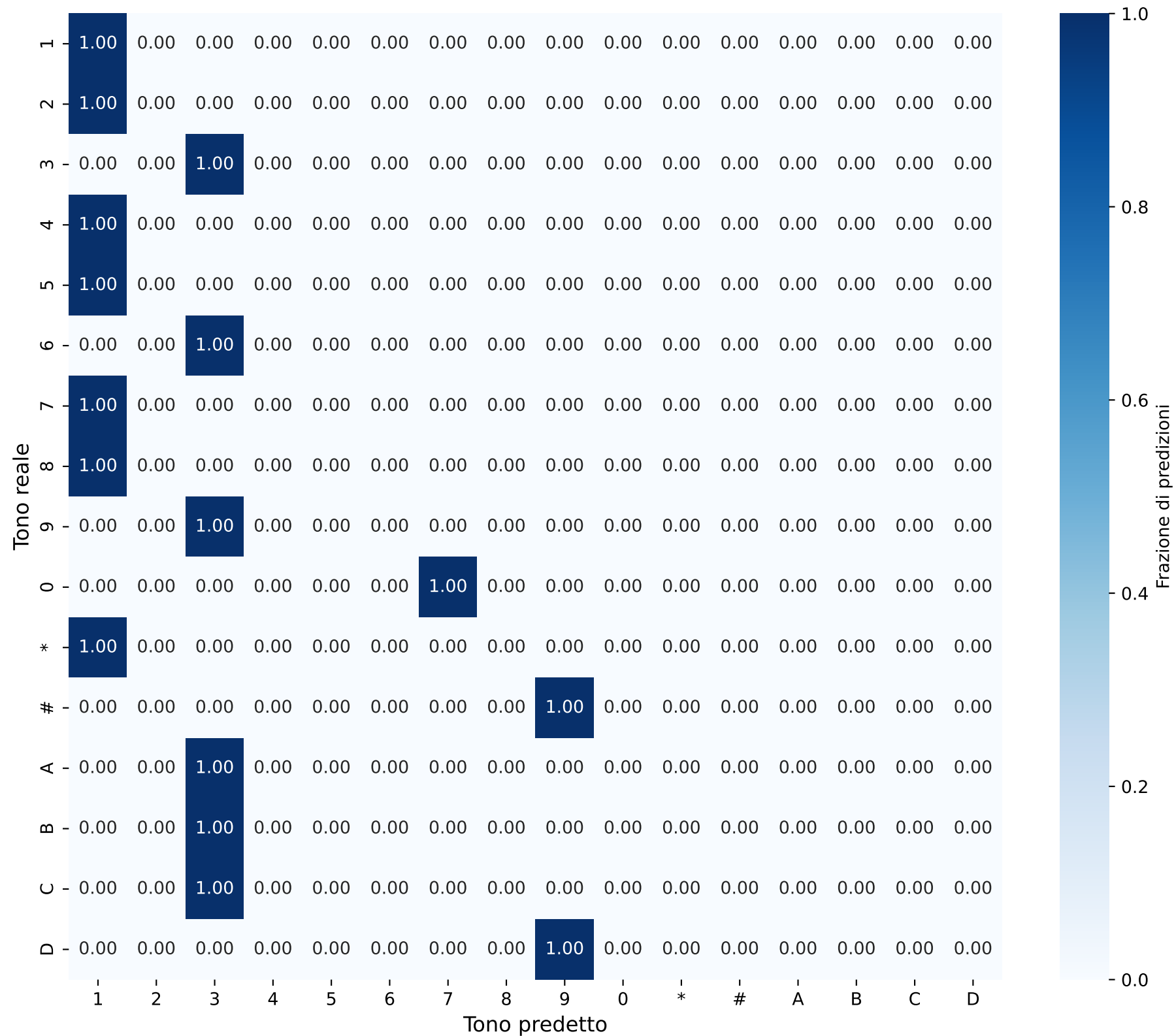
Matrice di Confusione - Singoli Toni Durata: 0.0037092697468885587s
