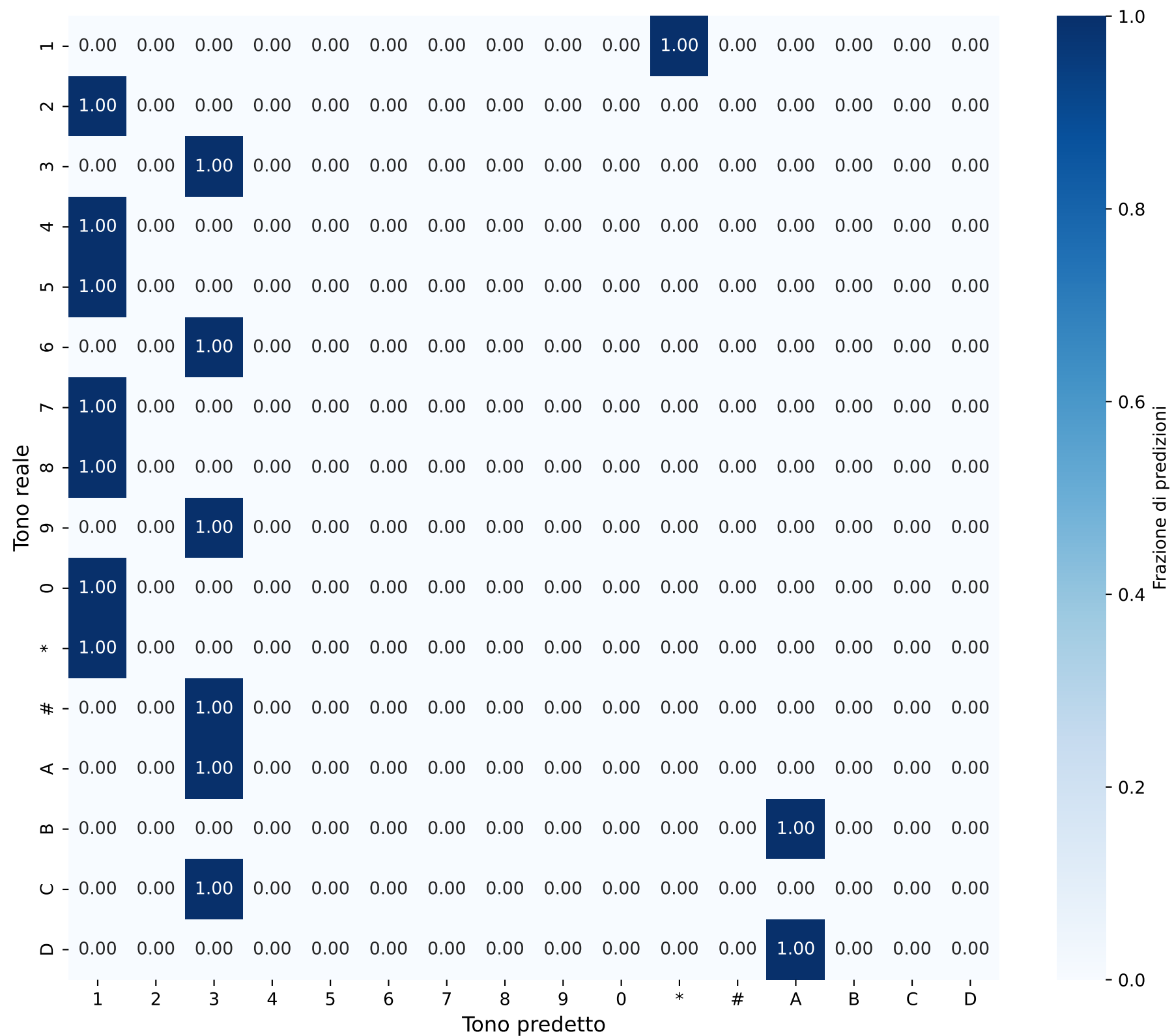
Matrice di Confusione - Singoli Toni Durata: 0.0044438415773643s
