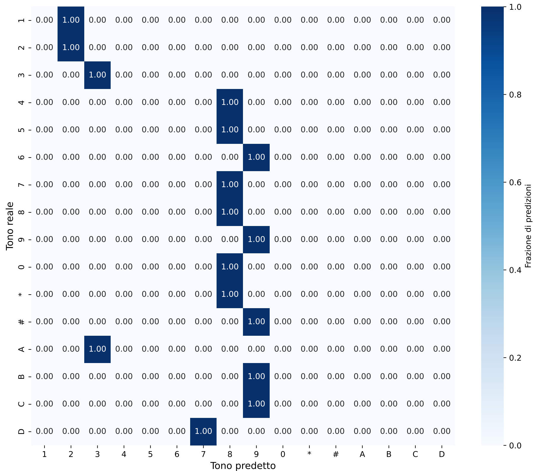
Matrice di Confusione - Singoli Toni Durata: 0.004543987642390772s
