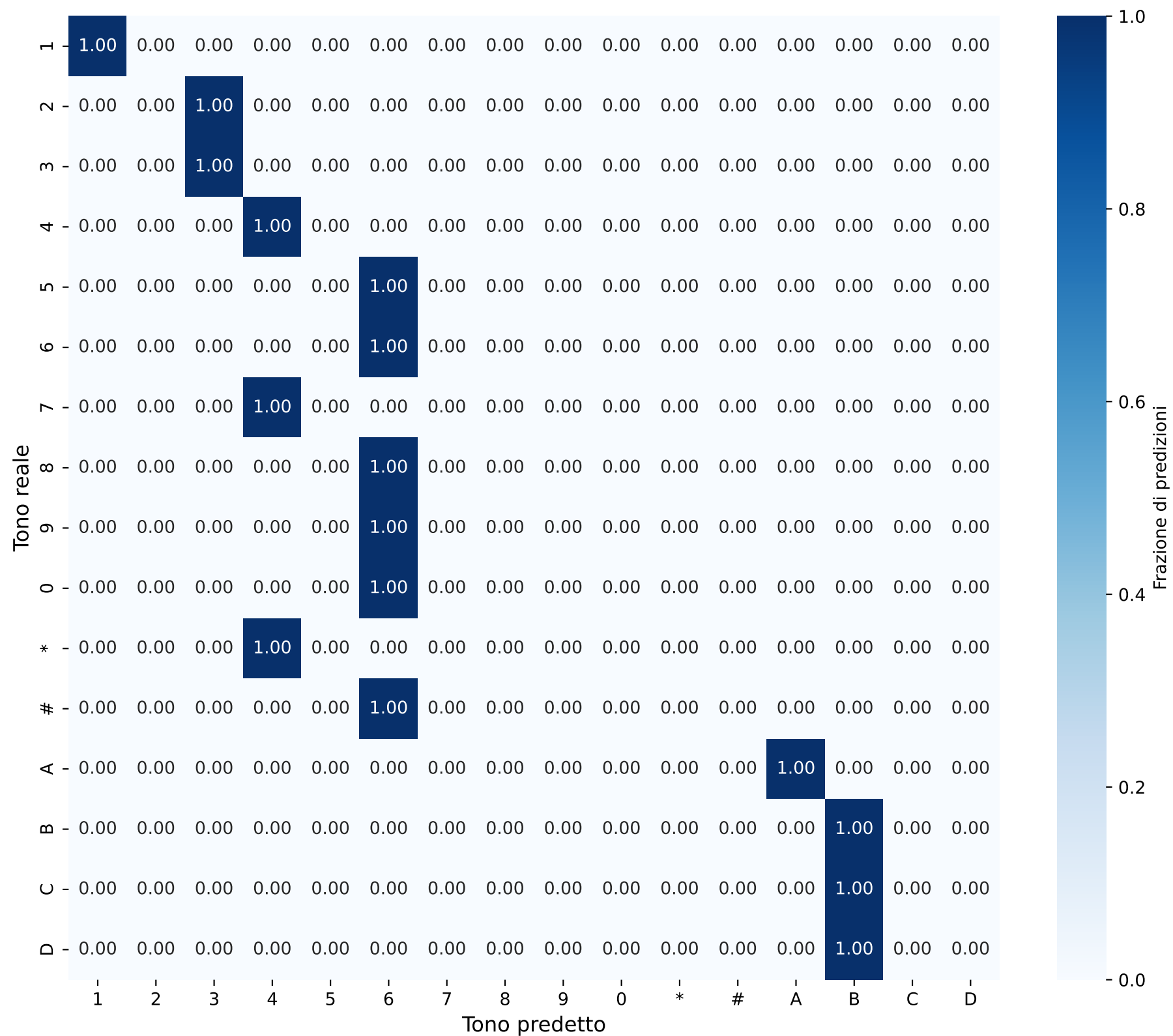
Matrice di Confusione - Singoli Toni Durata: 0.004813172483469571s
