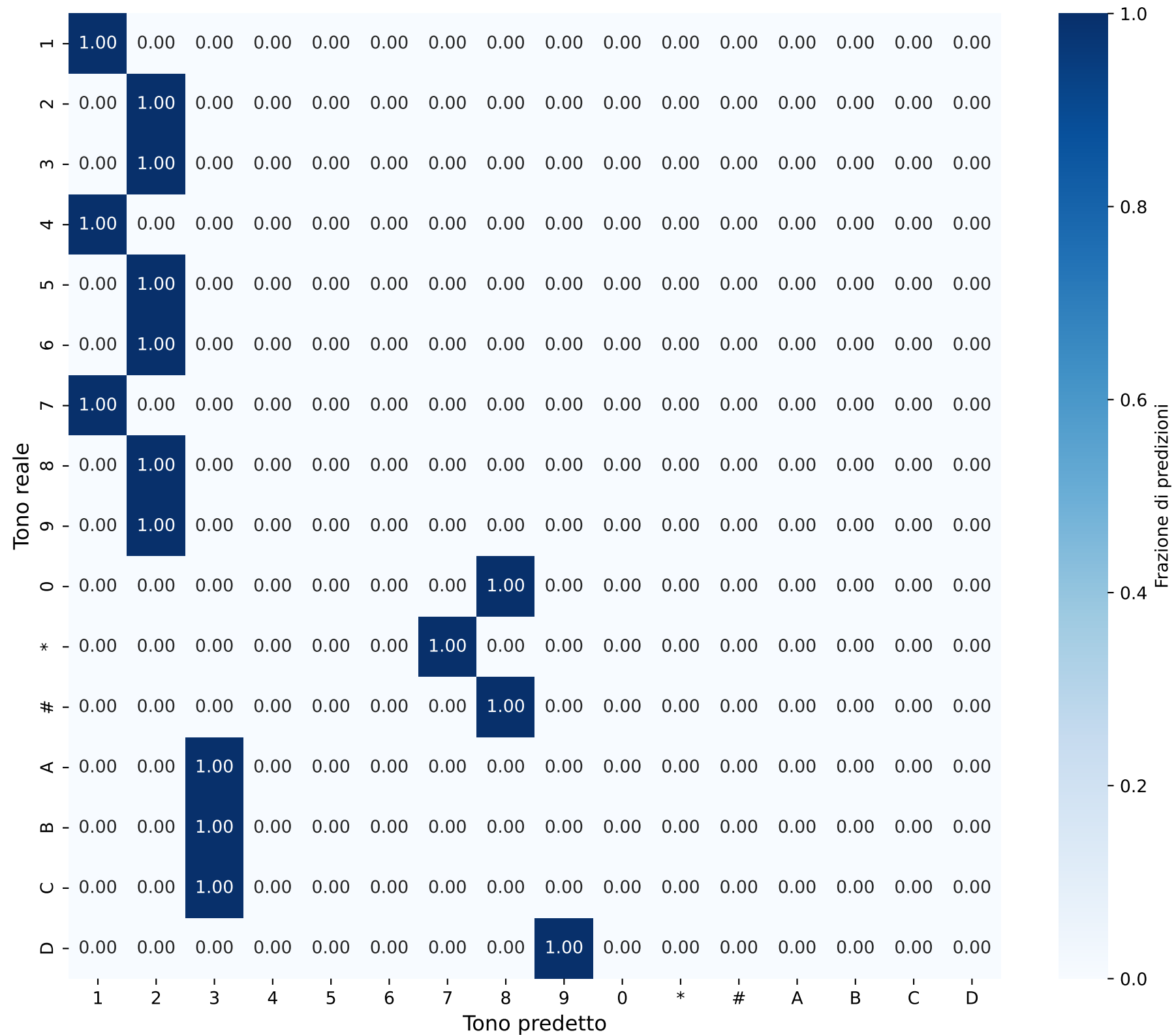
Matrice di Confusione - Singoli Toni Durata: 0.0048904256961953795s
