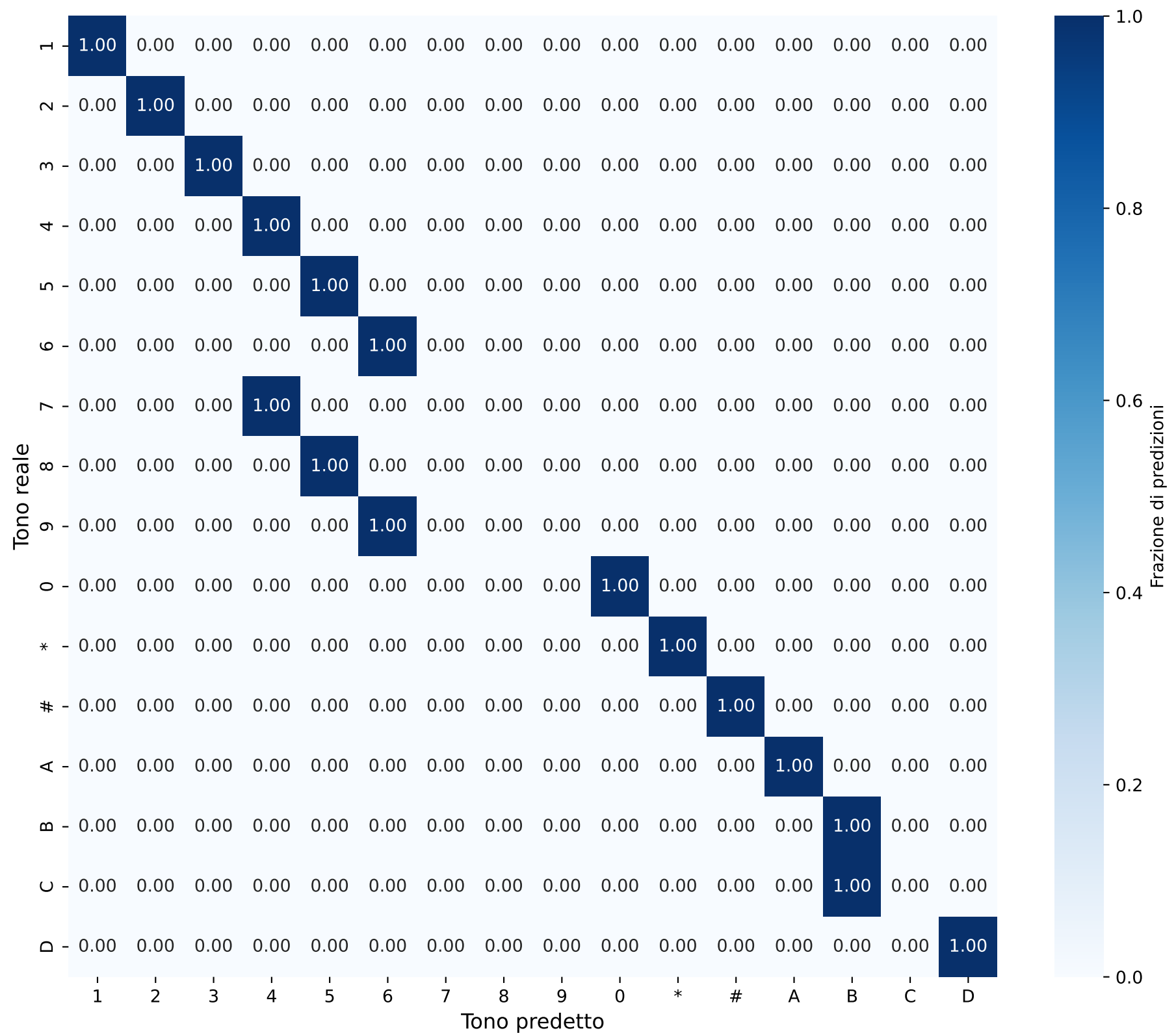
Matrice di Confusione - Singoli Toni Durata: 0.0075s
