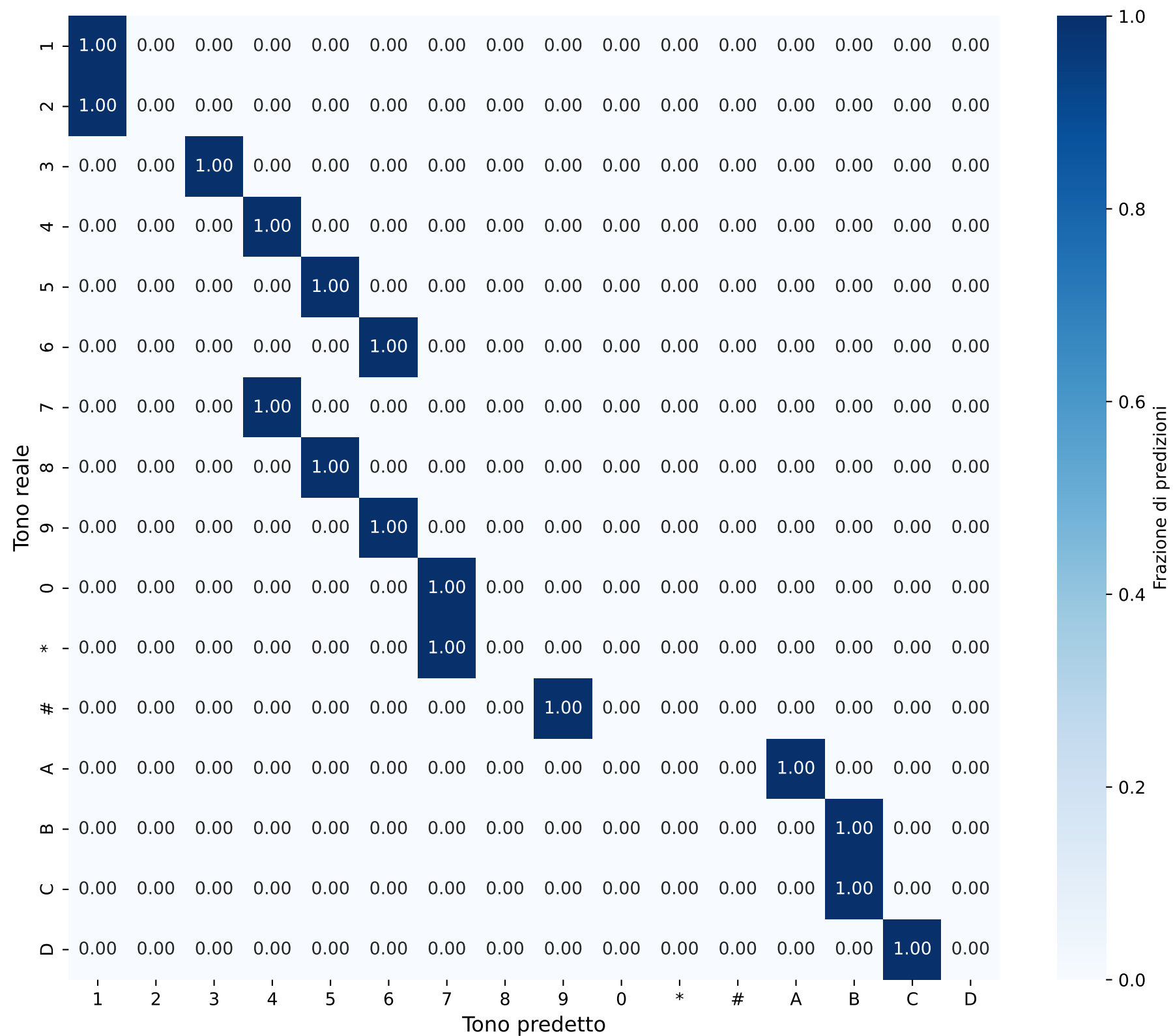
Matrice di Confusione - Singoli Toni Durata: 0.008452132819024976s
