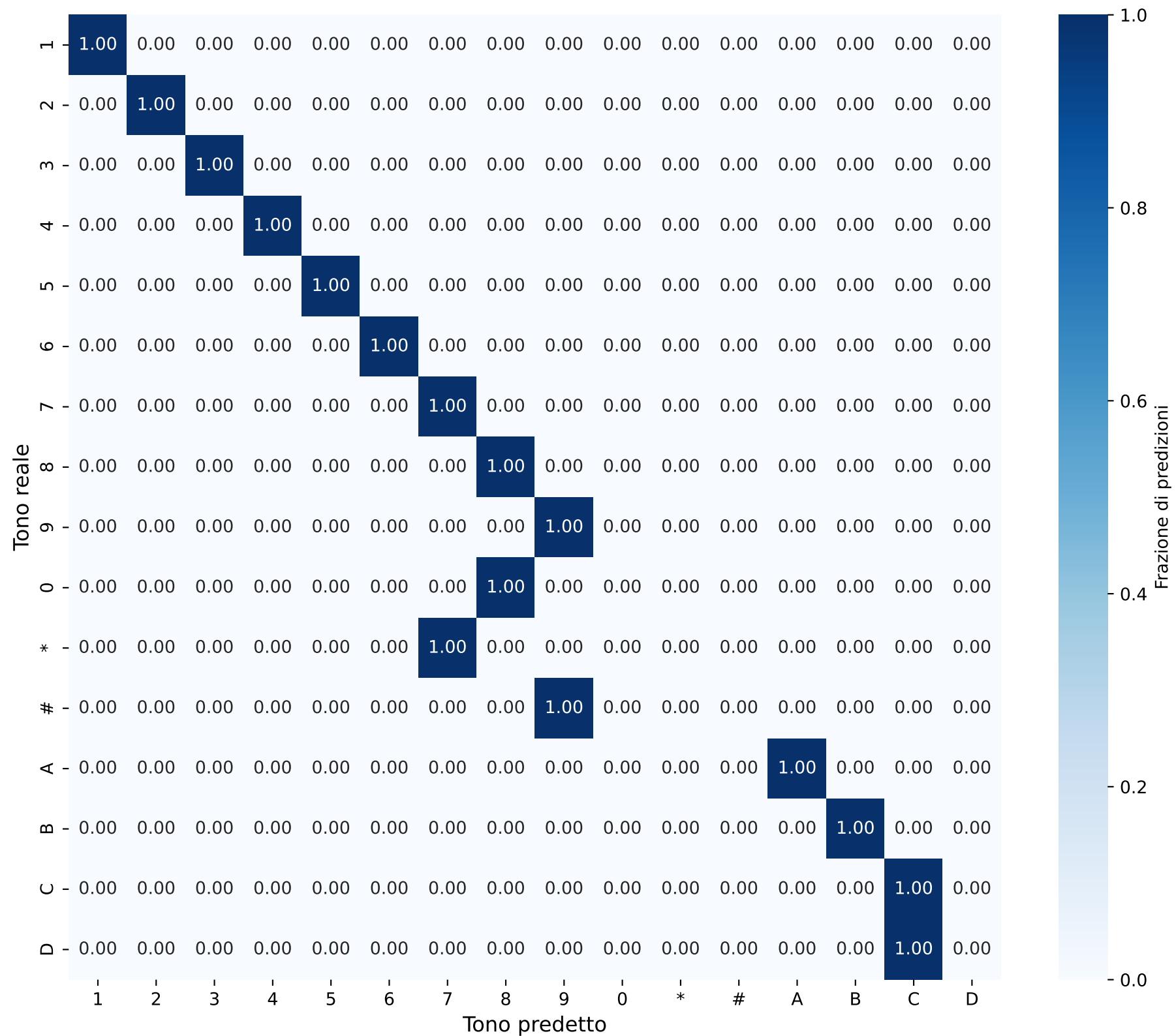
Matrice di Confusione - Singoli Toni Durata: 0.009116209203955908s
