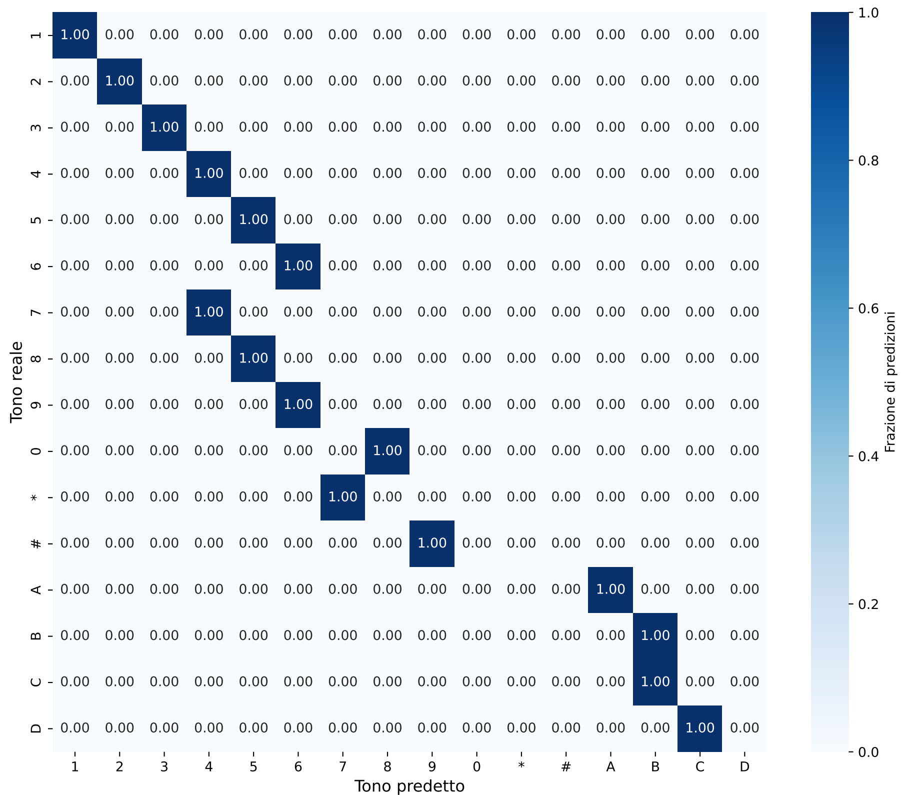
Matrice di Confusione - Singoli Toni Durata: 0.009686250859269968s
