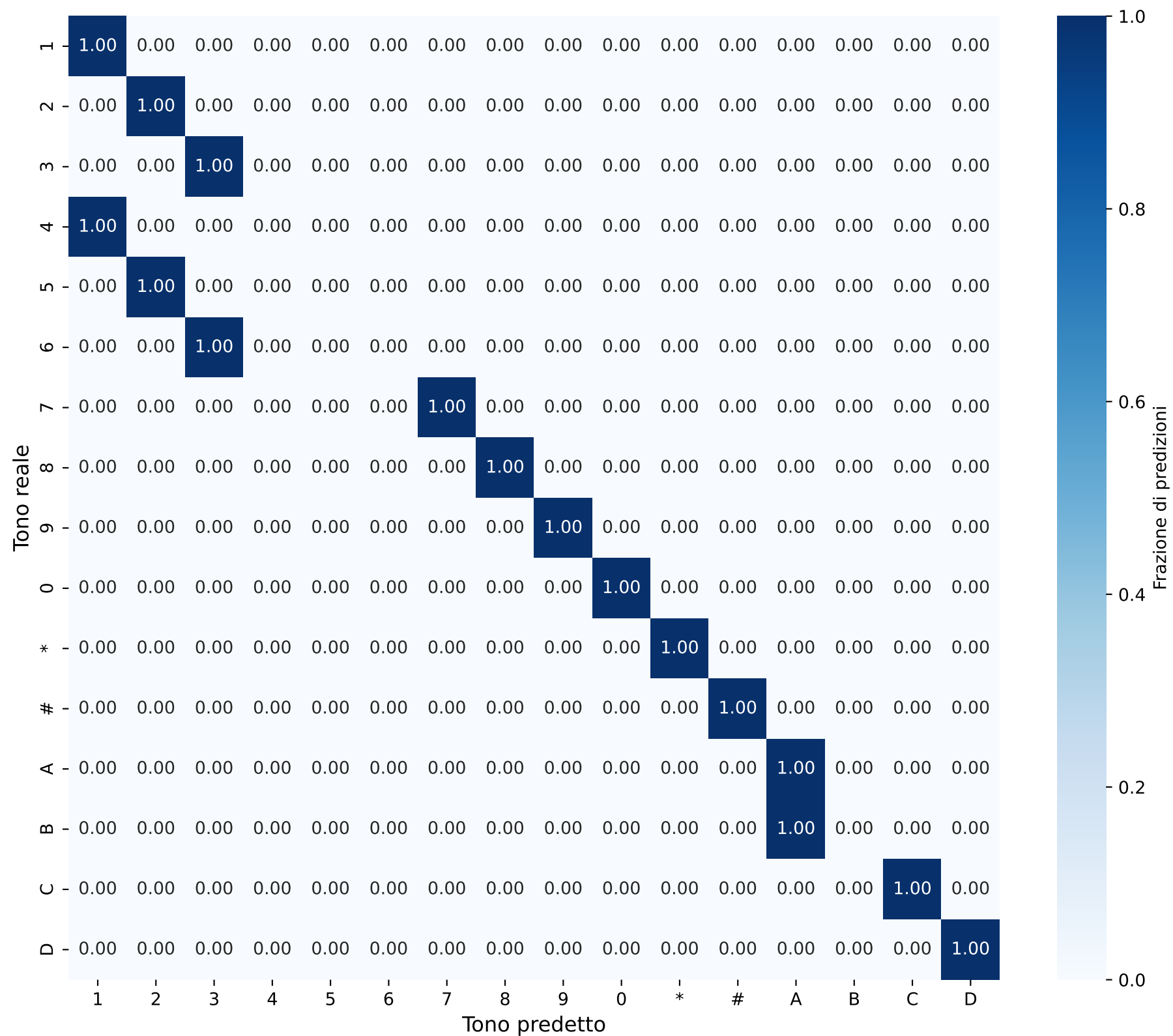
Matrice di Confusione - Singoli Toni Durata: 0.010384504693678718s
