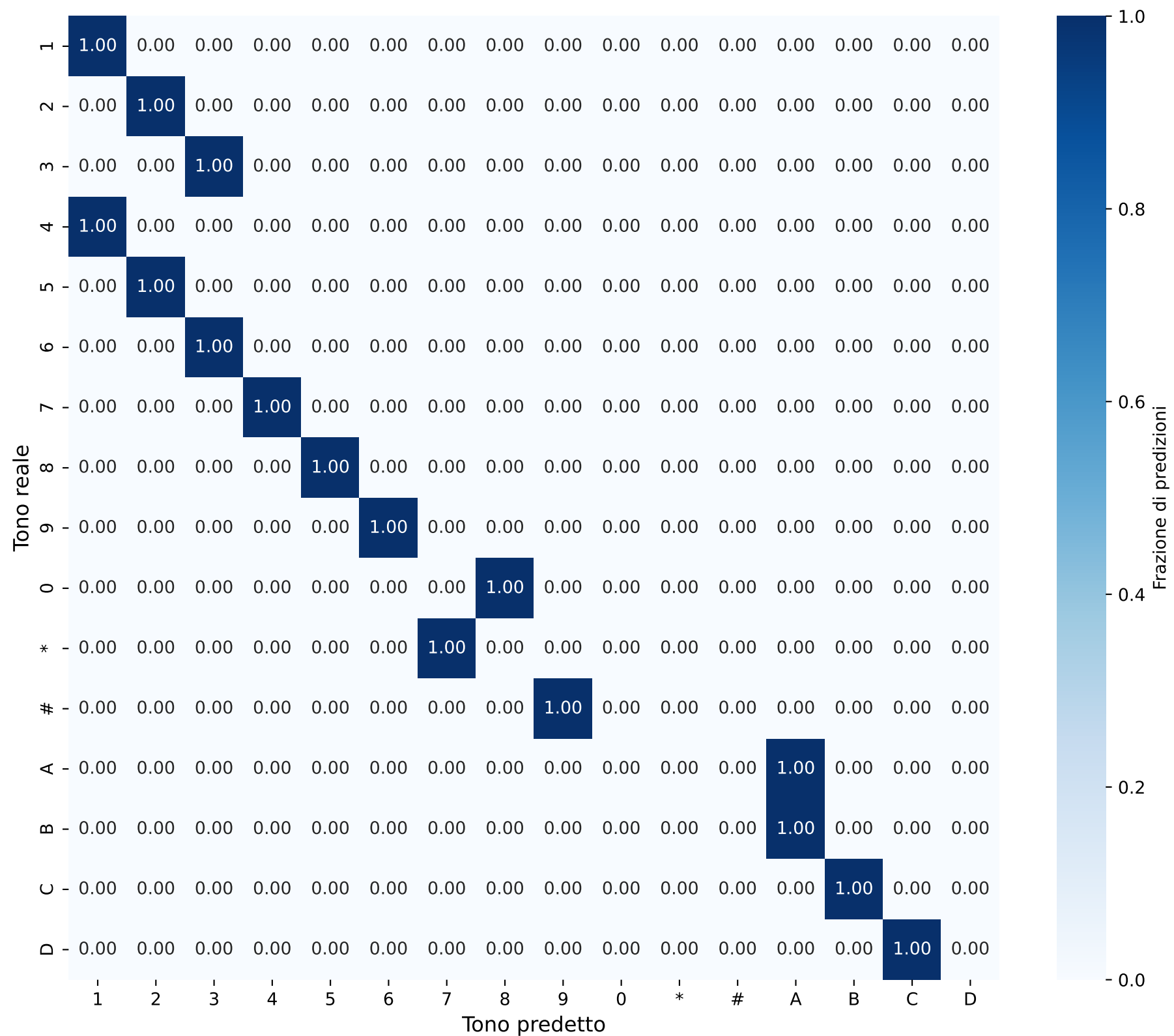
Matrice di Confusione - Singoli Toni Durata: 0.01069448800053393s
