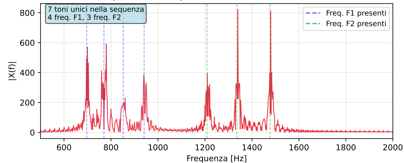
Spettro della sequenza - Risoluzione \Delta f = 20.0 Hz
