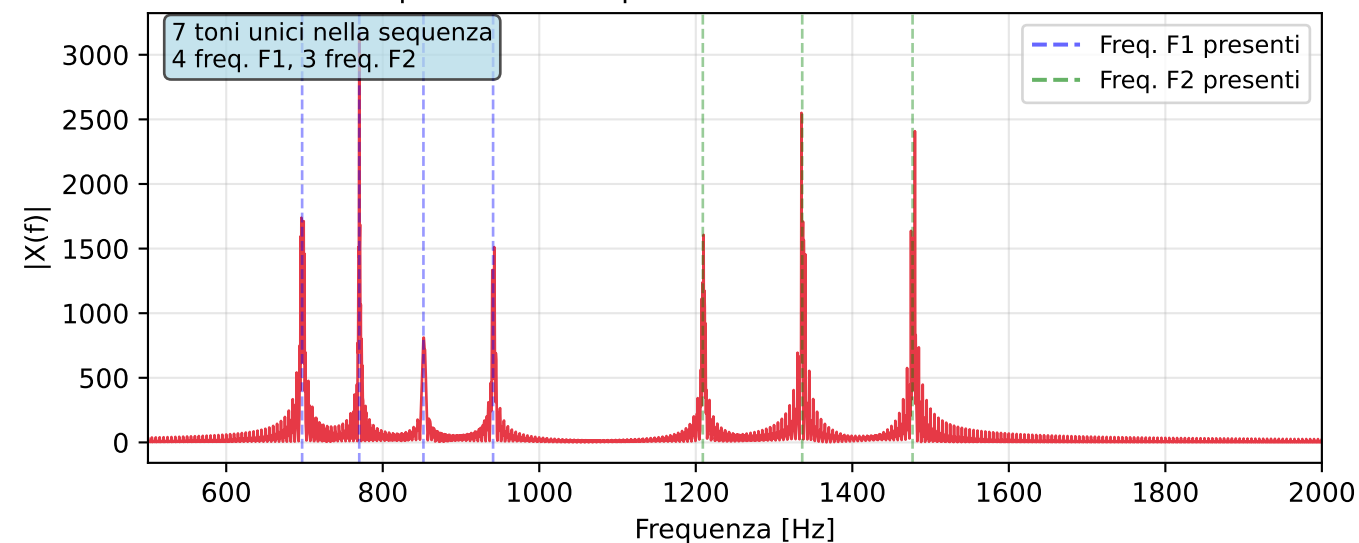
Spettro della sequenza - Risoluzione \Delta f = 5.0 Hz
