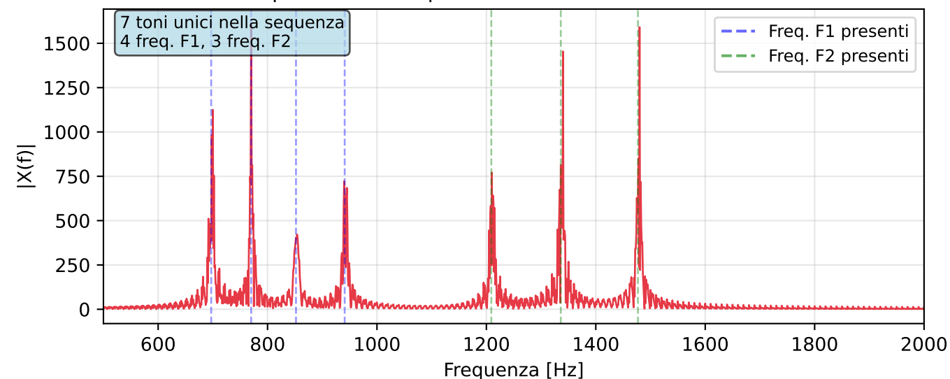
Spettro della sequenza - Risoluzione \Delta f = 10.0 Hz
