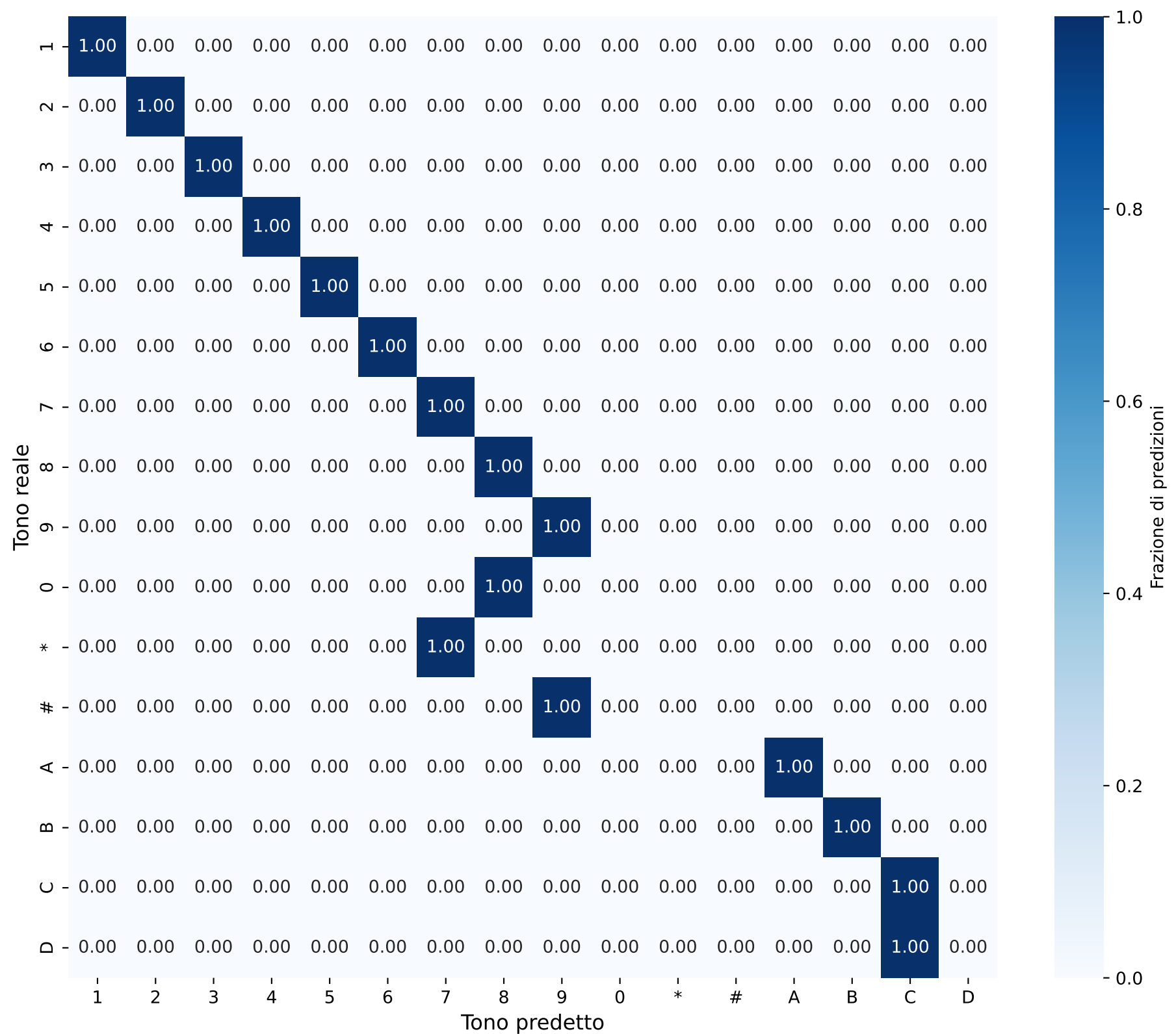
Matrice di Confusione - Sequenze Durata: 0.01s
