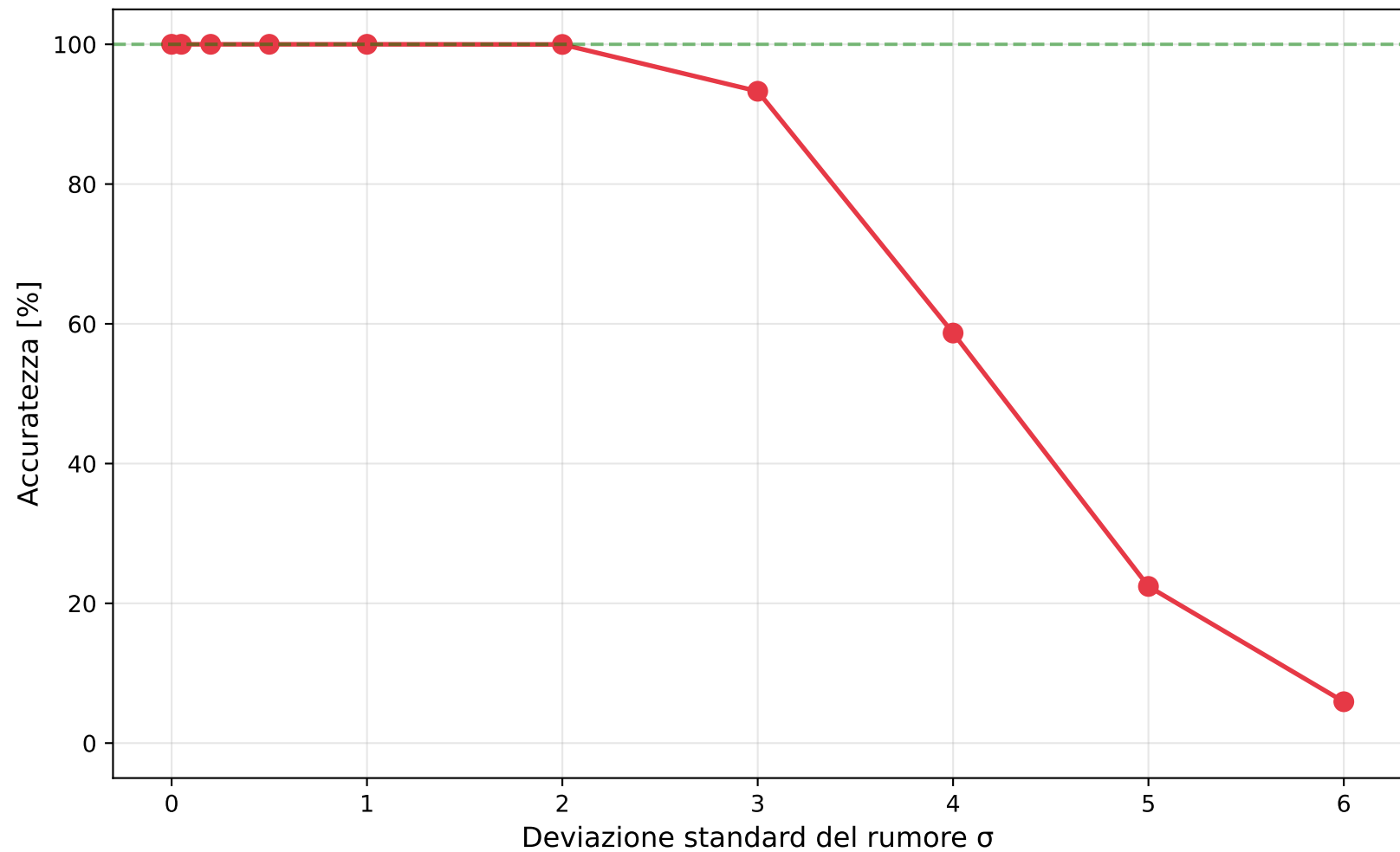
Accuratezza di riconoscimento DTMF in funzione del rumore
