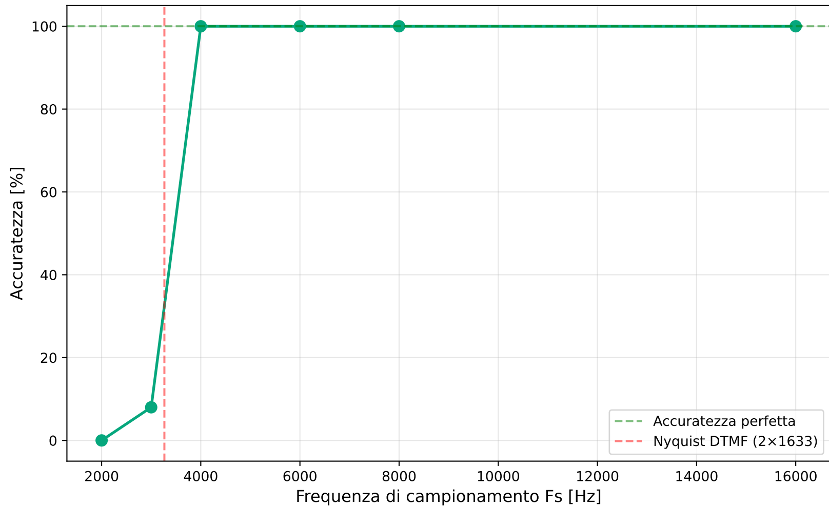
Accuratezza di riconoscimento DTMF vs Frequenza di campionamento
