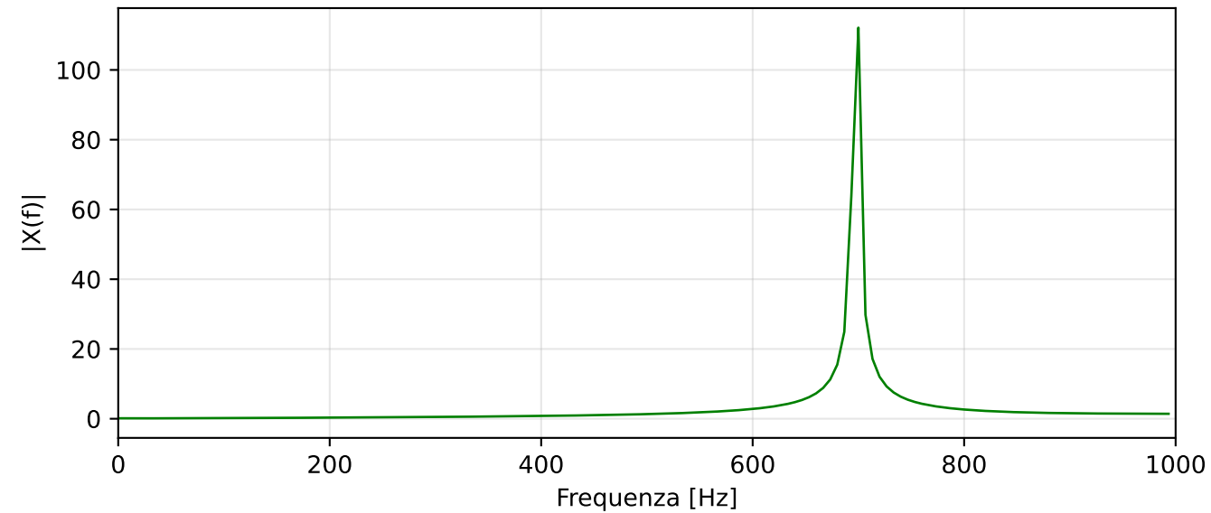
Spettro filtrato - F_s = 2000 Hz
