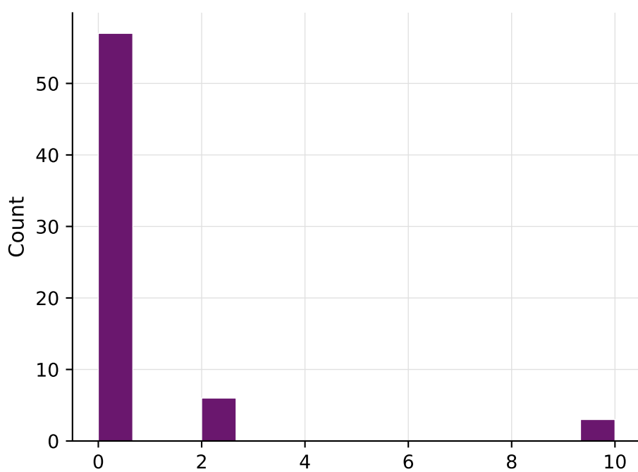
Ndata
