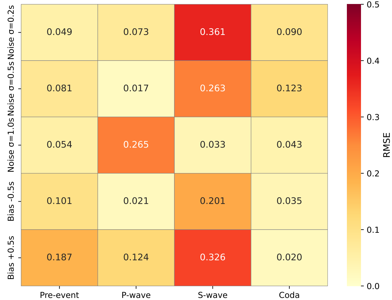
PHASENET
