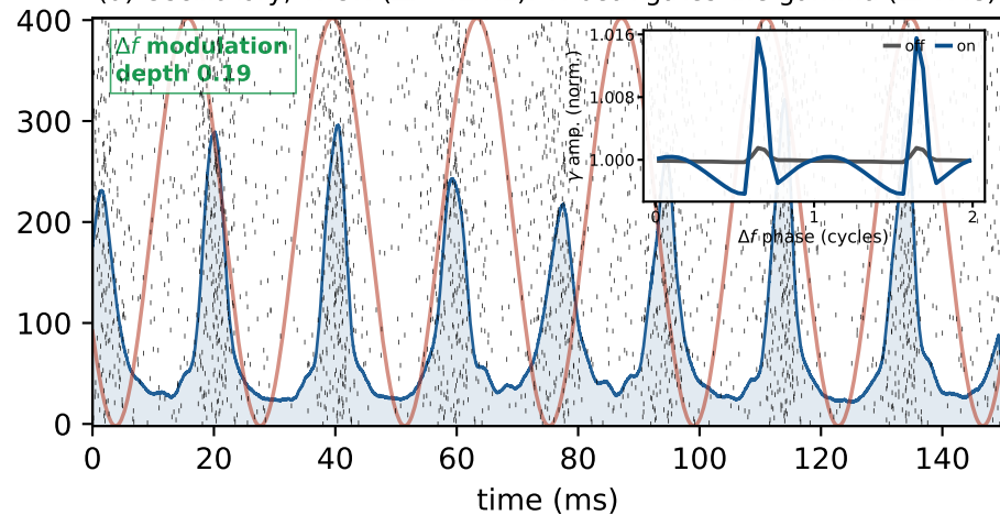
(d) Oscillatory, TI ON ( \Delta f=42 Hz): TI beat gates the gamma ( \Delta f -PAC)
