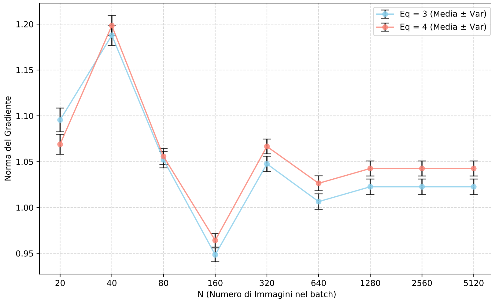
Norma del Gradiente vs N - Dataset: nwpu
