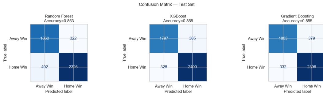
Figura 4.2: Matrici di confusione sul test set per il target home_win .
