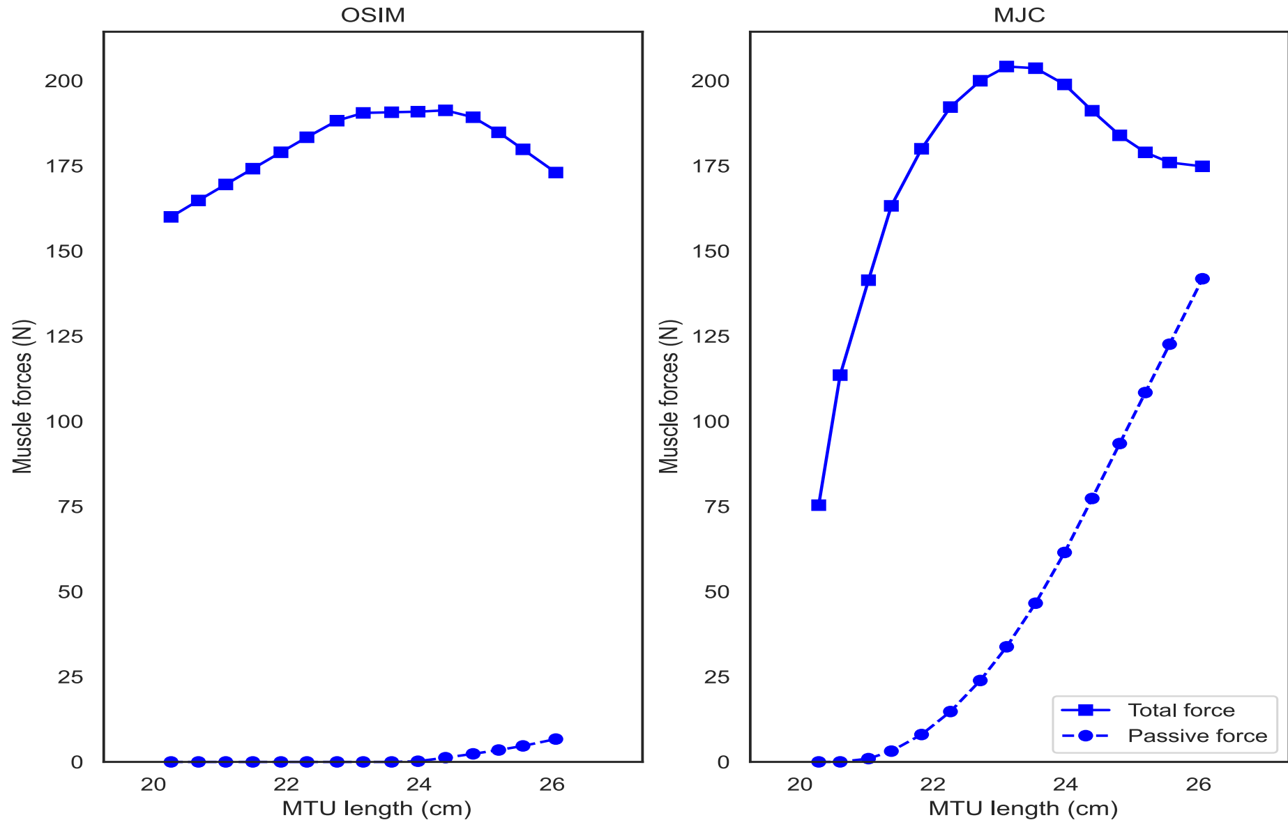
LFF_accesory_trochanter_flexor
