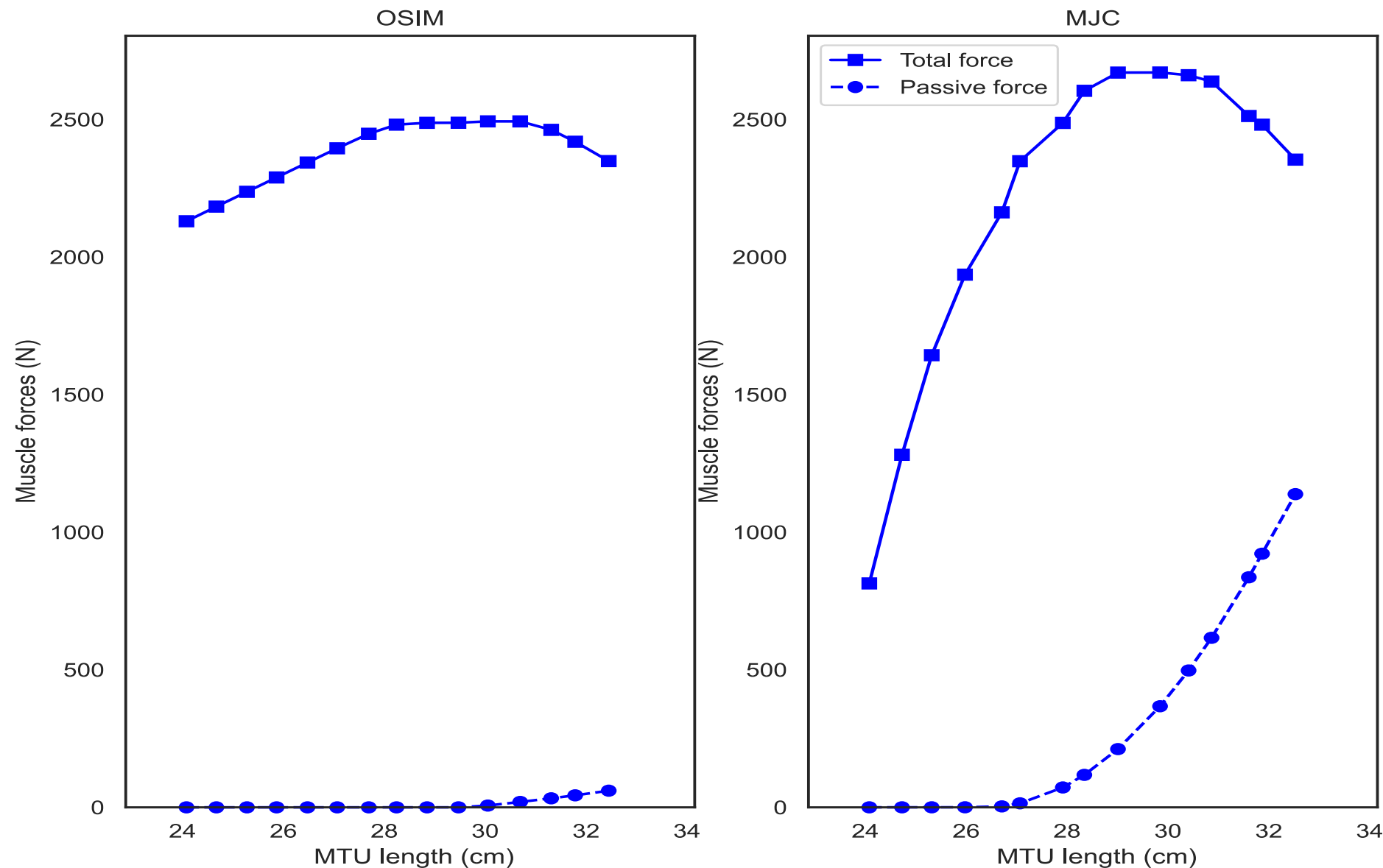
LFF_sterno-tergo-trochanter_extensor_b
