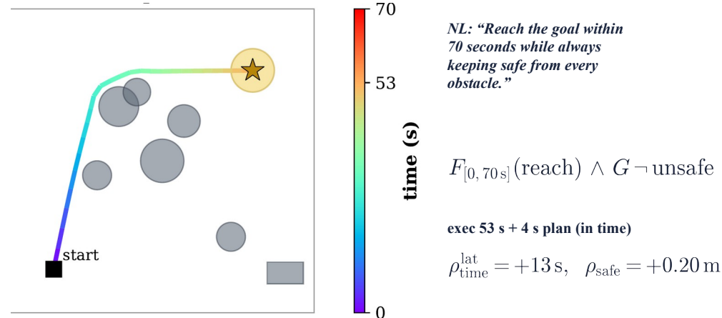
(c) TeLoGraF plan (no A*)
