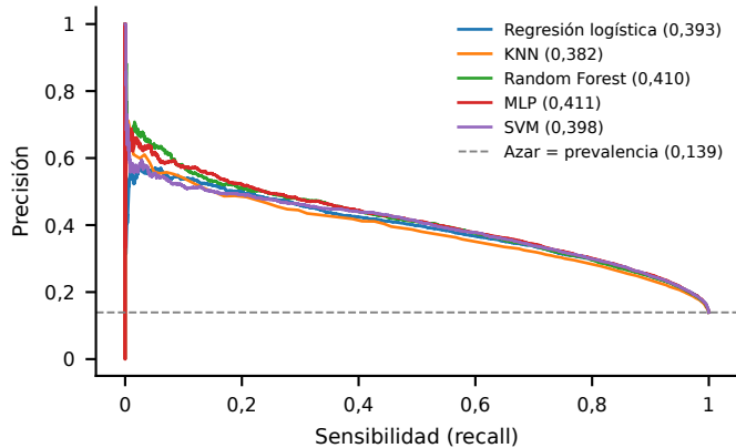
(b) Curvas precisión-sensibilidad (AUC-PR)
