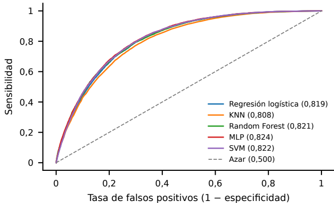
(a) Curvas ROC (AUC-ROC)
