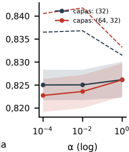
MLP
