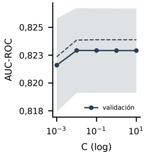
Regresión logística
