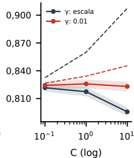
SVM
