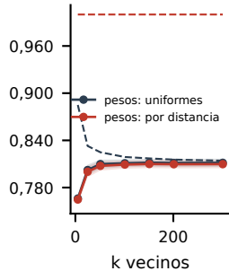
KNN
