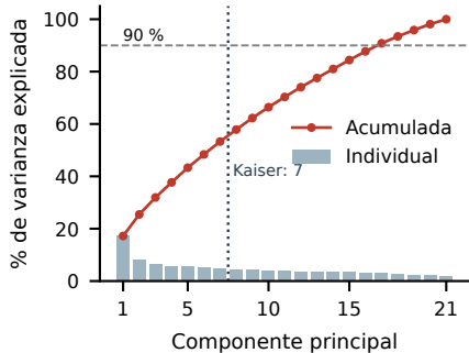
(a) PCA
