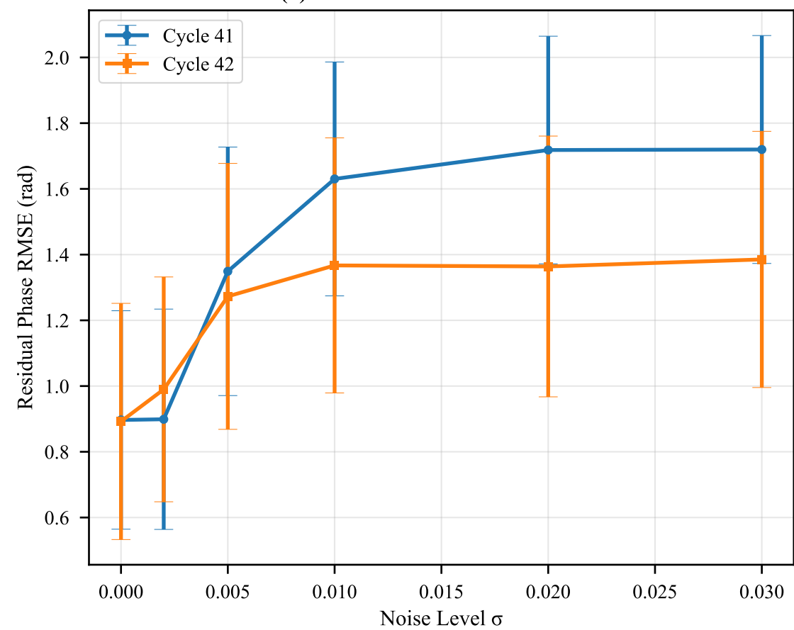
(d) Residual Phase RMSE vs Noise
