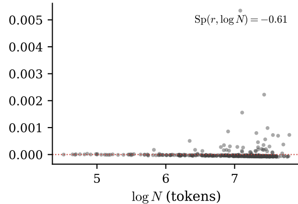
Curvature std
