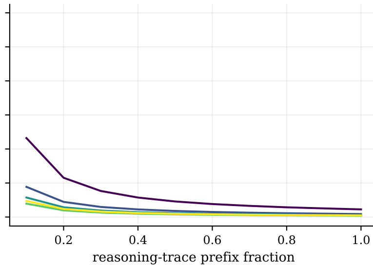
QwQ-32B
