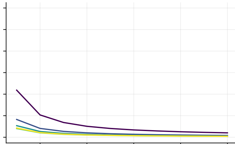
QwQ-32B
