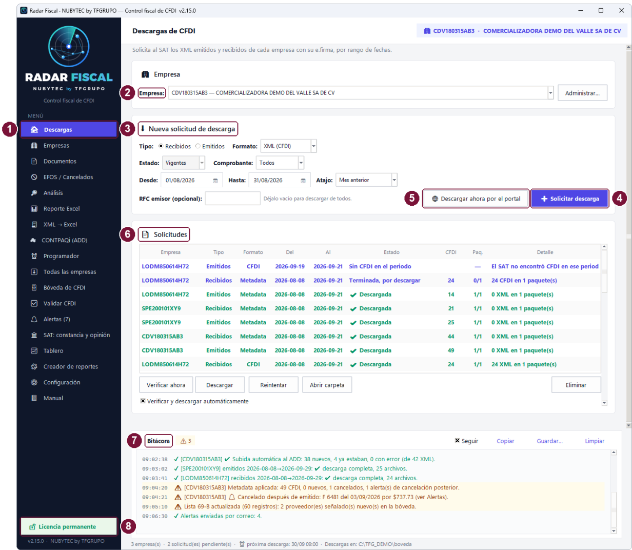
Pantalla principal: menú (1), empresa activa (2), nueva solicitud (3), solicitar (4), portal del SAT (5), solicitudes (6), bitácora (7) y licencia (8).
