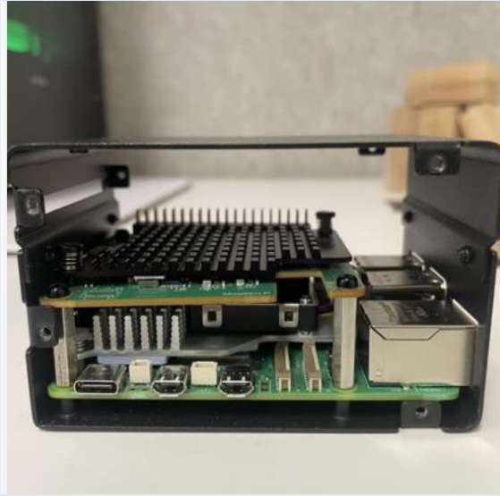
Raspberry Pi 5 16 GB + AI HAT+ 2 KKS 케이스 · 액티브 쿨러
