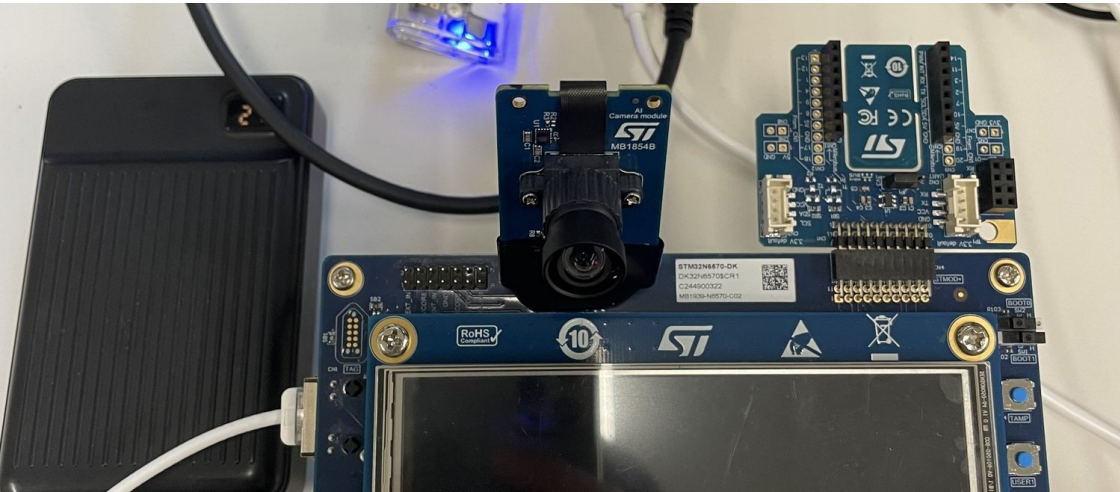
이 모델이 실제로 돌아가는 보드 — STM32N6570-DK 위의 AI 카메라 MB1854B 가 NPU 입력을 바로 공급한다
