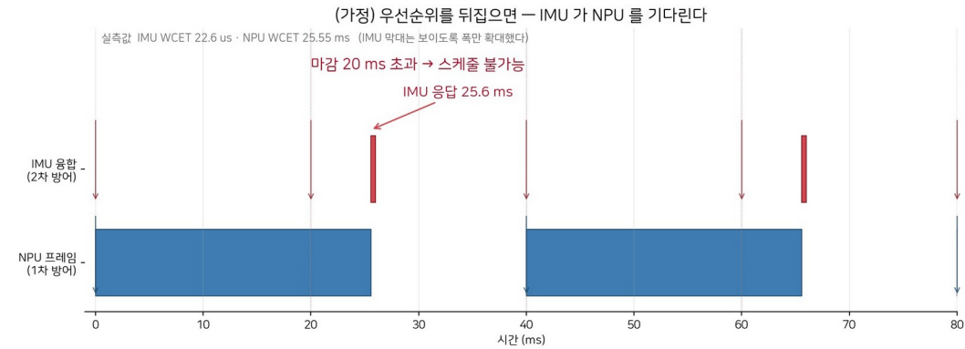
2번 변경의 근거 — 우선순위를 뒤집으면 NPU 추론(25 ms)이 IMU 주기(20 ms)를 막는다
