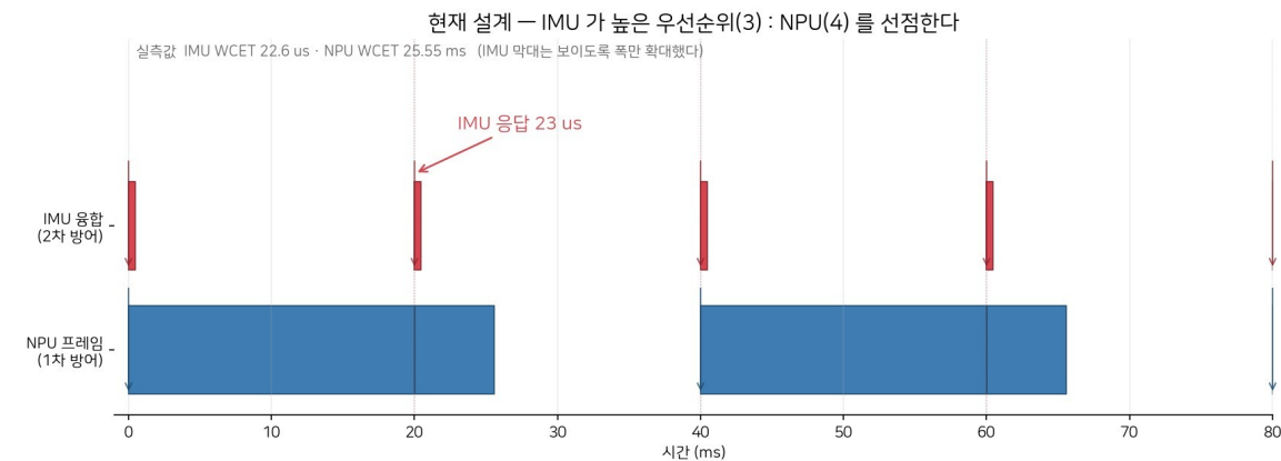
RM 스케줄 — IMU(우선순위 3)가 NPU(4)를 선점한다
