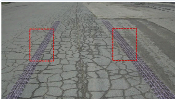
주행 영상에서 노면 영역만 잘라 패치로 쓴다
