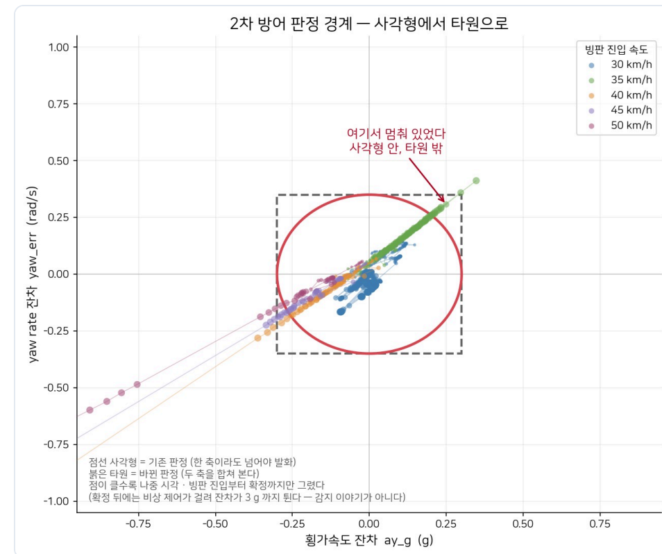
판정 경계 — 직사각형(점선) 대 타원(실선). 모서리에 걸리던 저속 구간이 타원에서 사라진다
