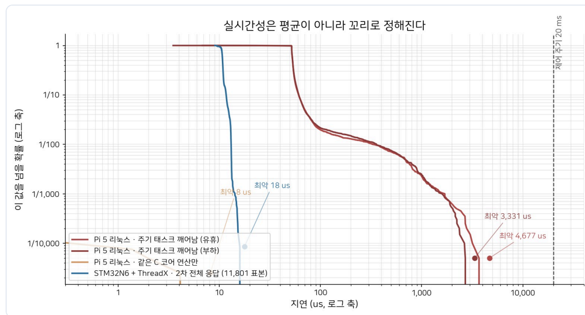
지연 분포 CDF — 리눅스는 꼬리가 길다
