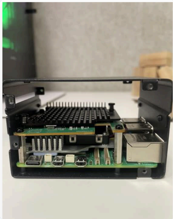
Pi 5 16 GB + AI HAT+ 2 (Hailo-10H) KKS 케이스 · 액티브 쿨러
