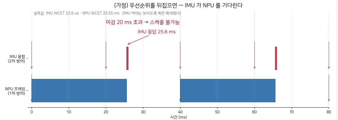
2번 변경의 근거 — 우선순위를 뒤집으면 NPU 추론(25 ms)이 IMU 주기(20 ms)를 막아 스케줄이 성립하지 않는다
