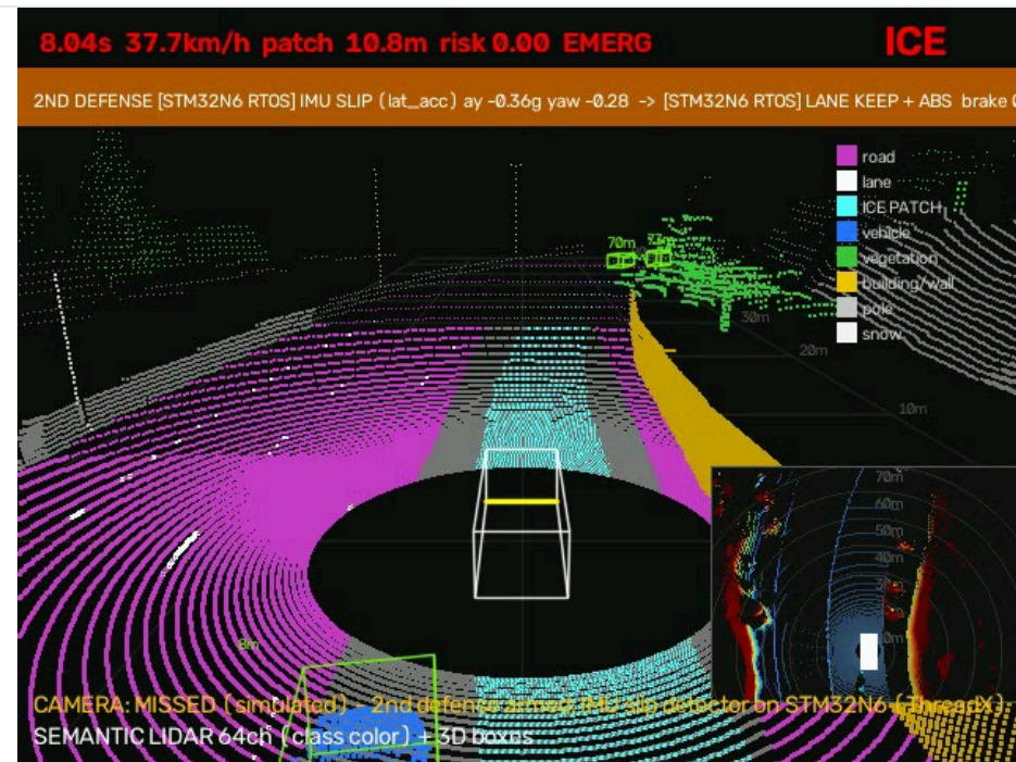
시맨틱 라이다 64채널 — 청록이 빙판 구간, 초록 상자가 차량 3D 박스. 미끄러짐 확정 순간
