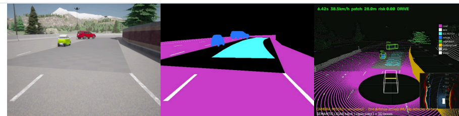
카메라 · 2D 분할 라벨 · 라이다 — 도로/차선/빙판/차량 라벨을 자동 생성한다 (AI Hub 형식 참고)
