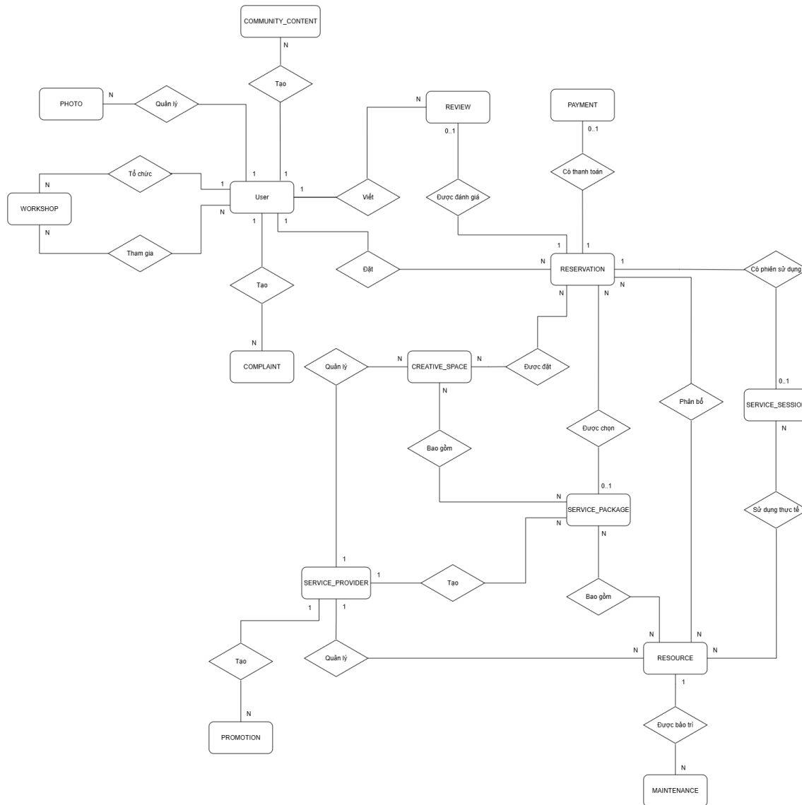
FIGURE 2.1. Sơ đồ Thực thể - Mối kết hợp (ERD) mức quan niệm hoàn chỉnh
