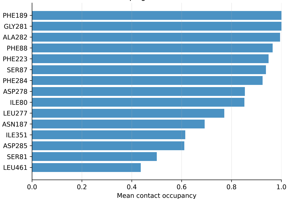
CYP1B1: top ligand-contact residues
