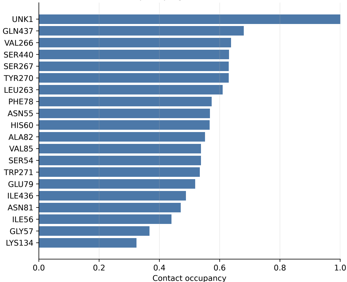
SGLT2 rep1 top ligand-contact residues
