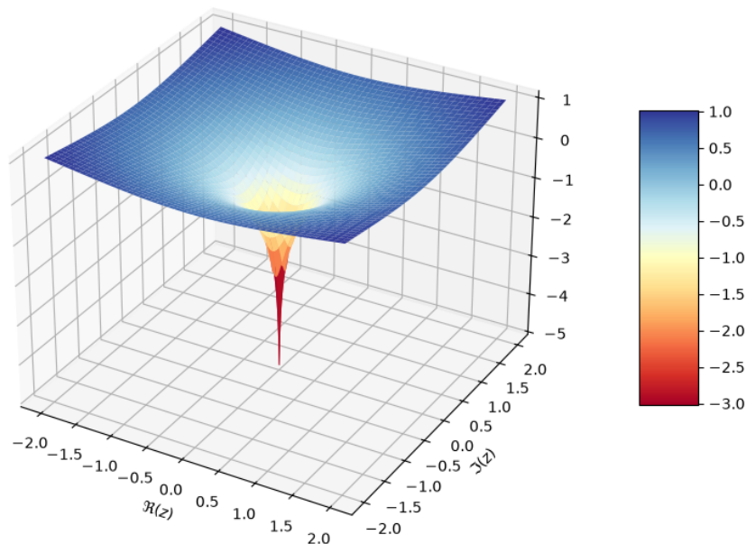
Figure 1: Parte real del logaritmo .
