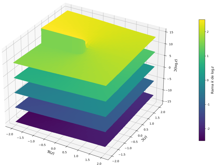
Figure 3: Superficie de Riemann del logaritmo.
