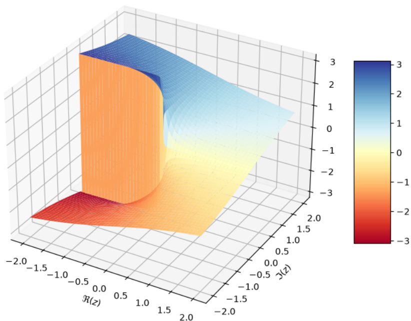
Figure 2: Parte imaginaria del logaritmo.
