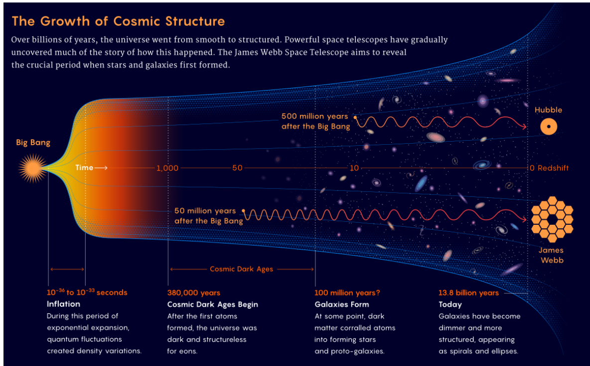
Figura 4: El crecimiento de la estructura cósmica. Créditos: Samuel Velasco (Quanta Magazine)
