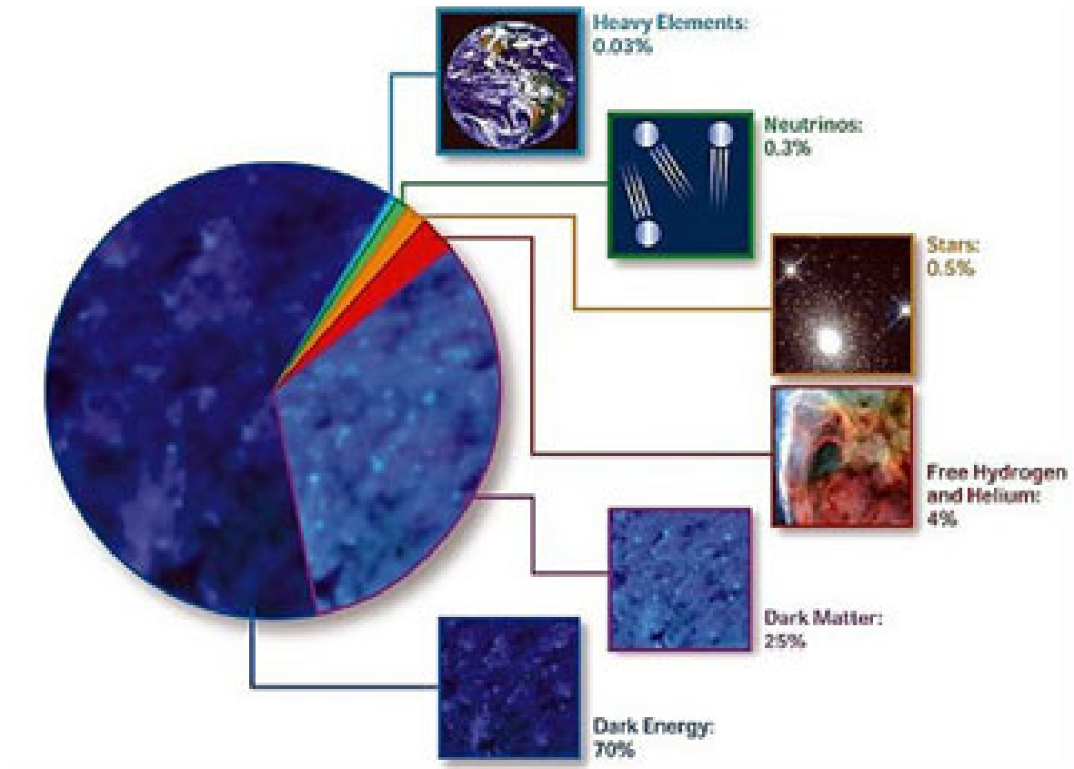
Figura 3: Composición del universo.
