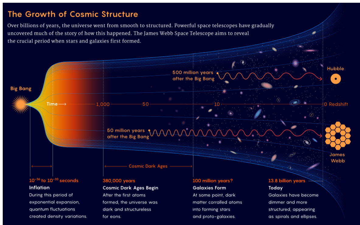
Figure 4: El crecimiento de la estructura cósmica. Créditos: Samuel Velasco (Quanta Magazine)
