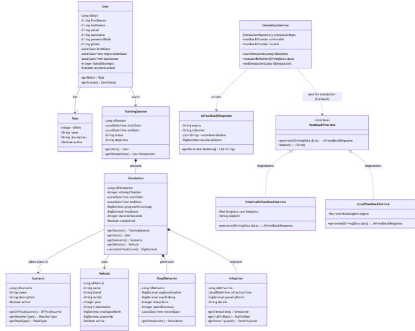
Figura 2.3: Diagrama de Clases UML para los componentes principales. Fuente: Elaboración propia.
