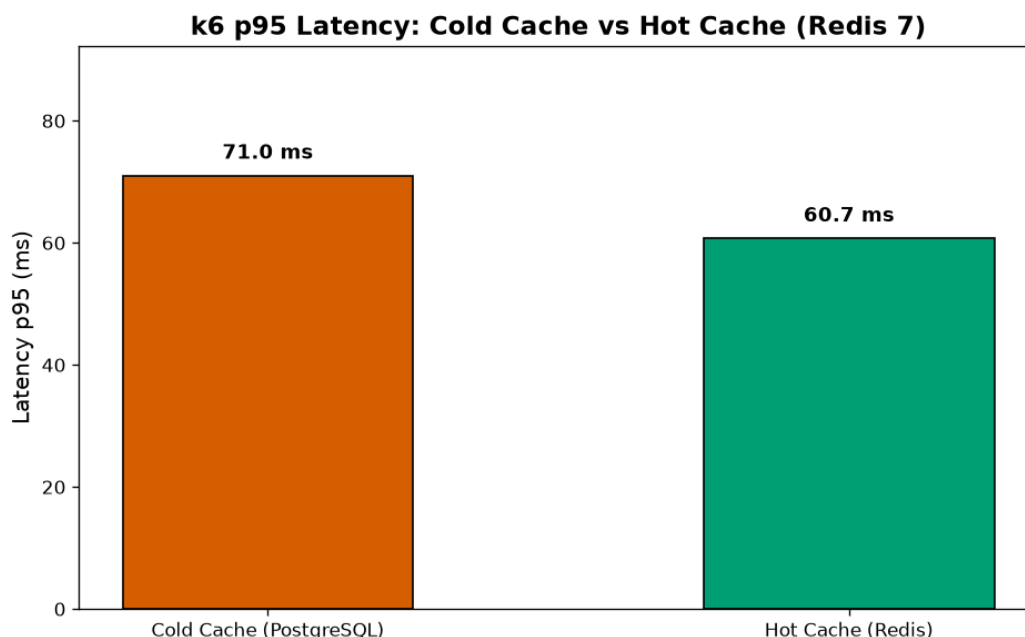
Figura 8.1: Distribución de latencia comparativa de las ejecuciones de k6. Fuente: Elaboración propia.
