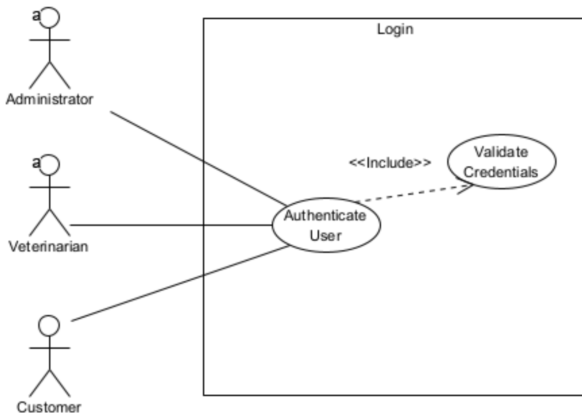
Ilustración 4. Caso de uso Inicio de sesión
