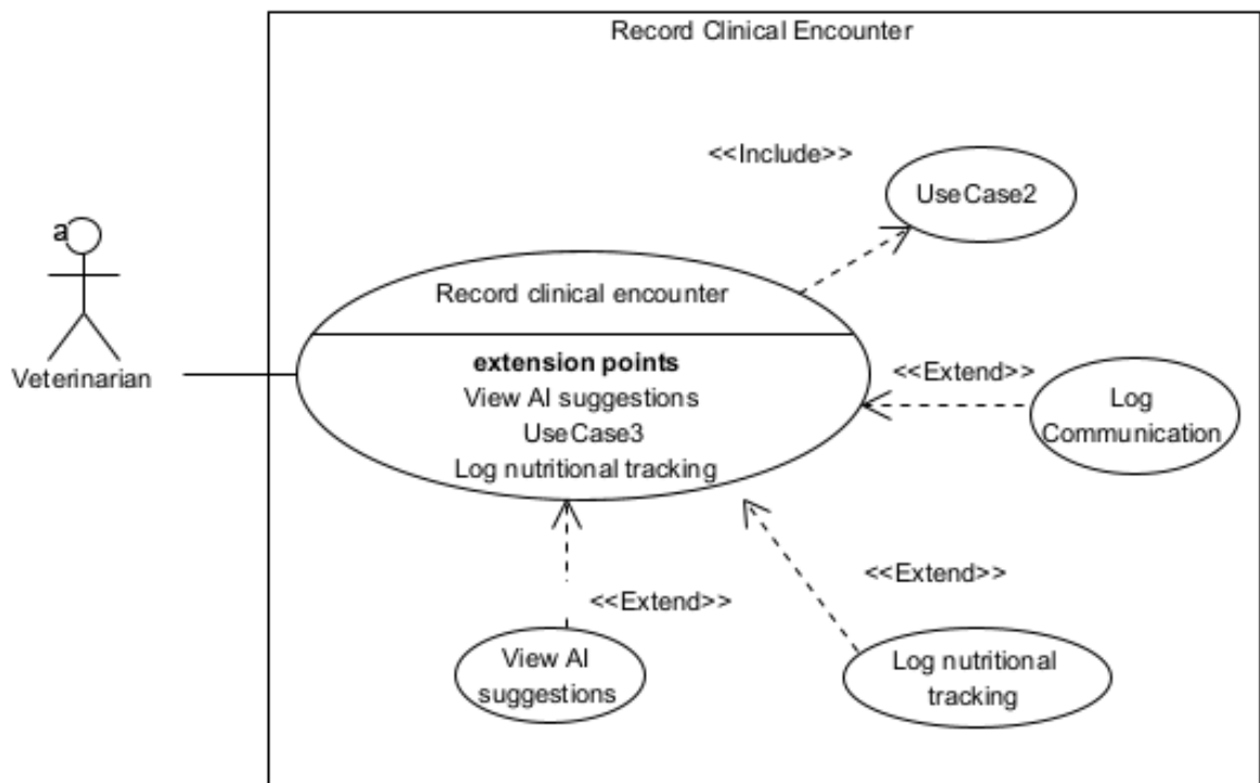
Ilustración 5. Caso de uso Registrar atención clínica
